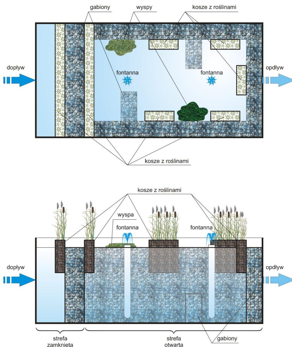
Rys. 51 Propozycje zmian w projektowanym zbiorniku mających na celu intensyfikację procesów mechanicznego i biochemicznego podczyszczania wód Potoku Królewskiego i spływów opadowych
