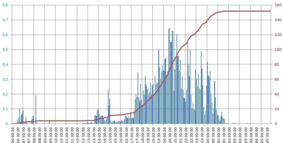
Rys. 6 Natężenie opadu [mm/min] oraz krzywa skumulowana opadu [mm] w dniach 14-15 lipca 2016 r.; źródło: http://www.klimat.ug.edu.pl/?page_id=5092
