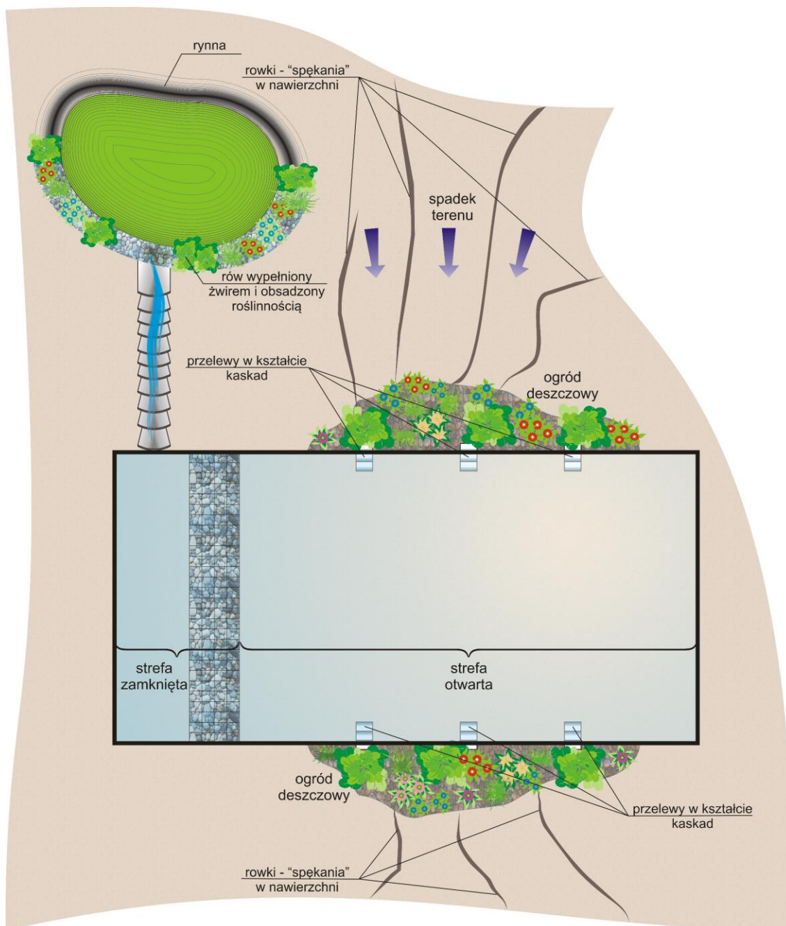
Rys. 52 Propozycja podczyszczania wód opadowych przed odprowadzeniem do projektowanego zbiornika
