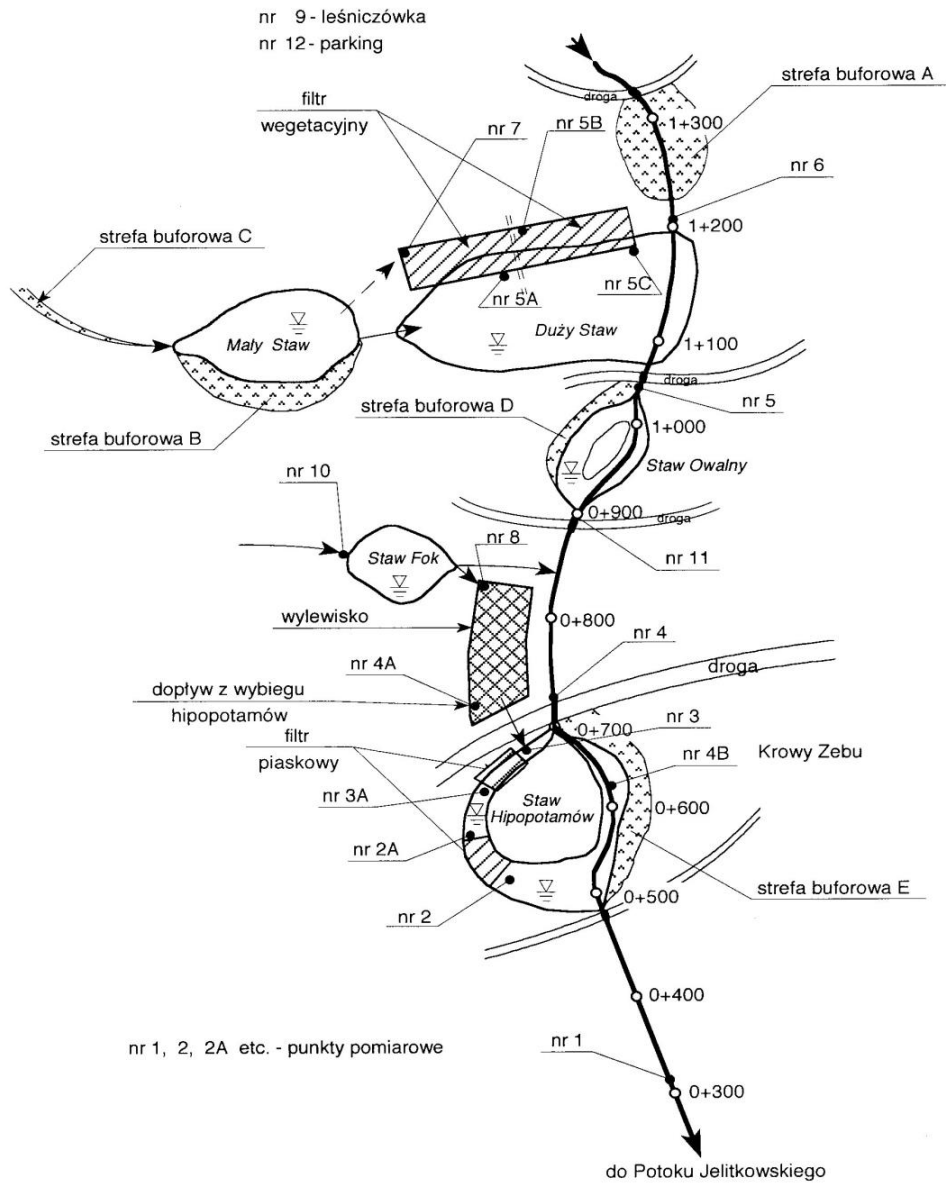
Rys. 45 Schemat systemu hydrofitowego zastosowanego w ogrodzie zoologicznym w Gdańsku w celu ochrony wód Potoku Rynarzewskiego.
